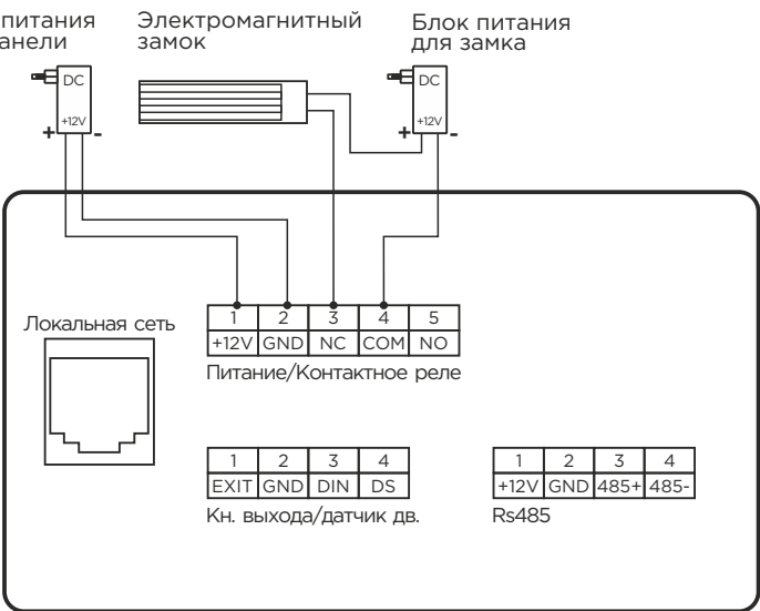
Схема подключения электромеханического замка при внешнем источнике питания для замка. Схема подключения электромагнитного замка с использованием внешнего блока питания для замка.
